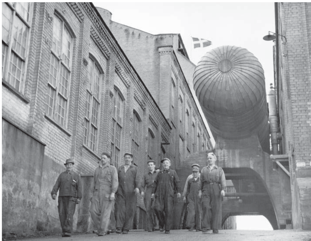
Nensjö sulfatfabrik, ångackumulator enl. Ruths. Bilden är tagen vid ett skiftbyte 1961. SCA:s bildarkiv.
